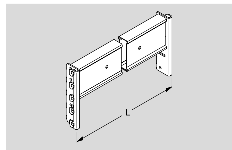
Traverse oben ITDL 120x40 für Plattenregal Profil 120x40 mm, mit Aushebesicherungen und Löcher für Unterteilungsrohre
