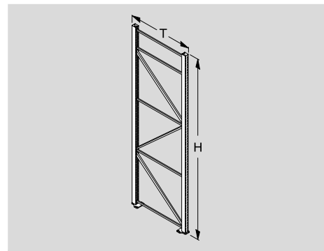
Ständer CG 70x80 für Plattenregal aus C-Profil 70x80 mm, Anlieferung zerlegt (inkl. Schrauben)
