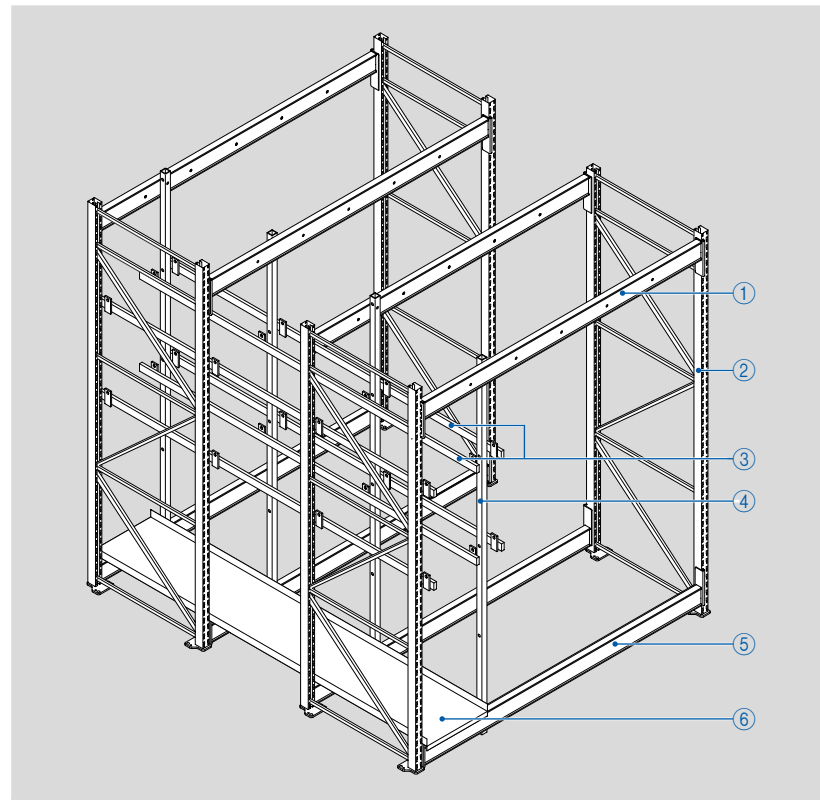
Ständer CG 70x80 für Plattenregal aus C-Profil 70x80 mm, Anlieferung zerlegt (inkl. Schrauben)
