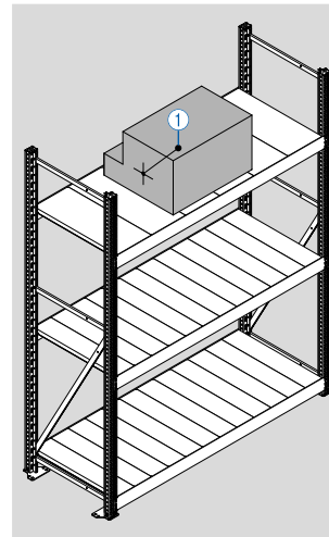
① Lastschwerpunkt
